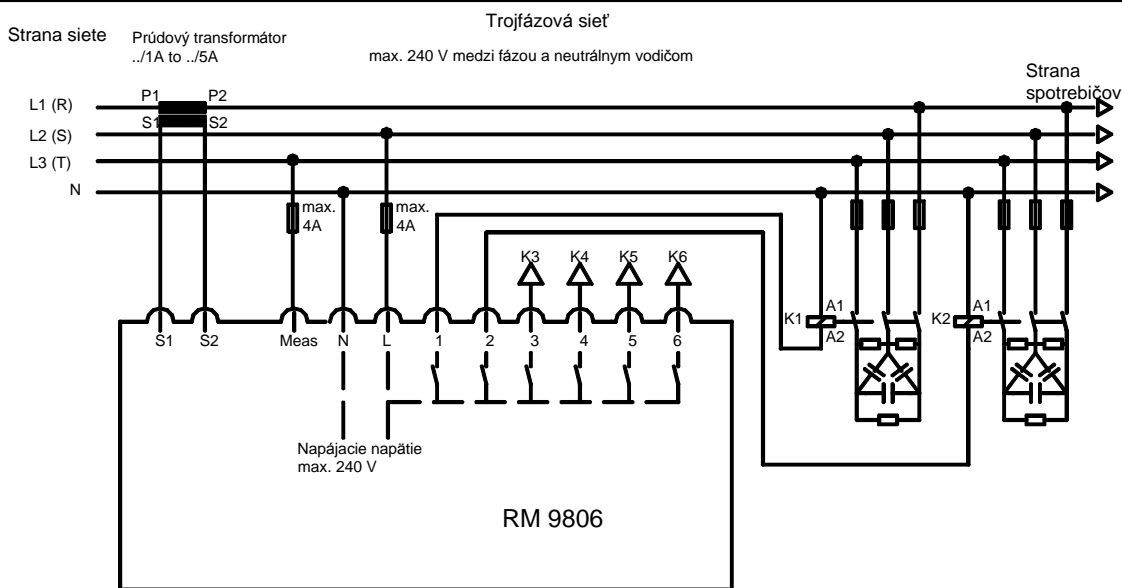
Obr. 4: Rozšírené pripojenie
