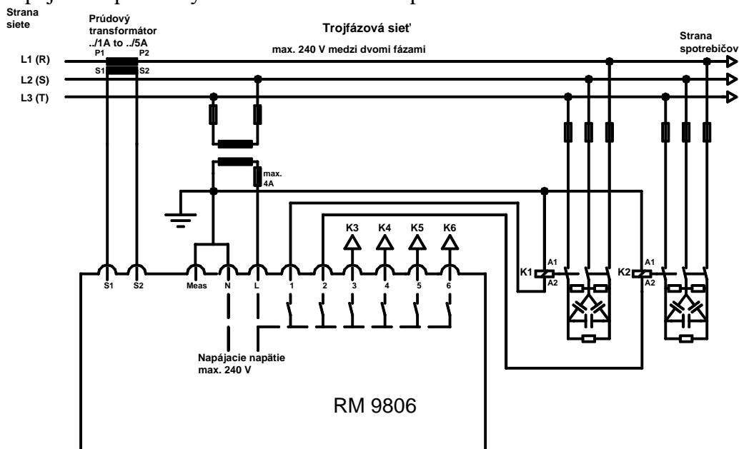
Obr. 5: Pripojenie s prevodným transformátorom napätia.
