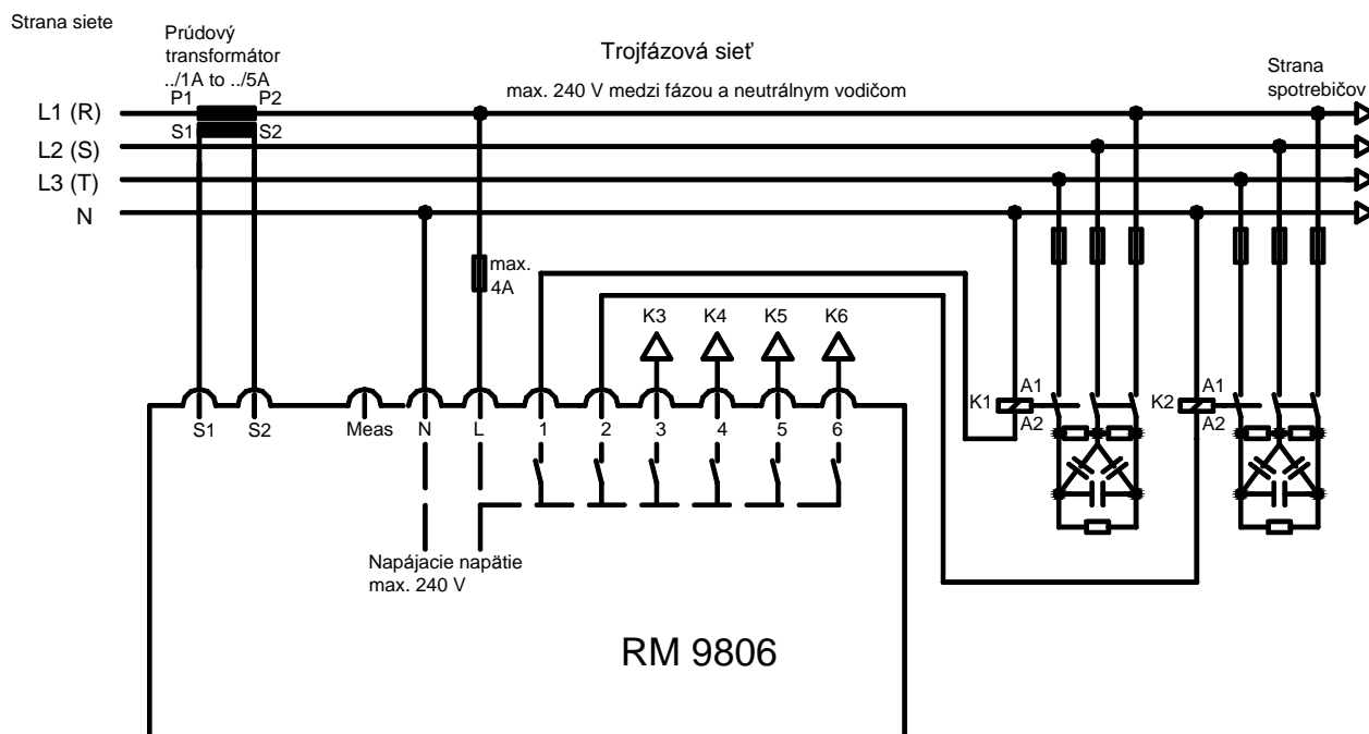
Obr. 3: Štandardné zapojenie
